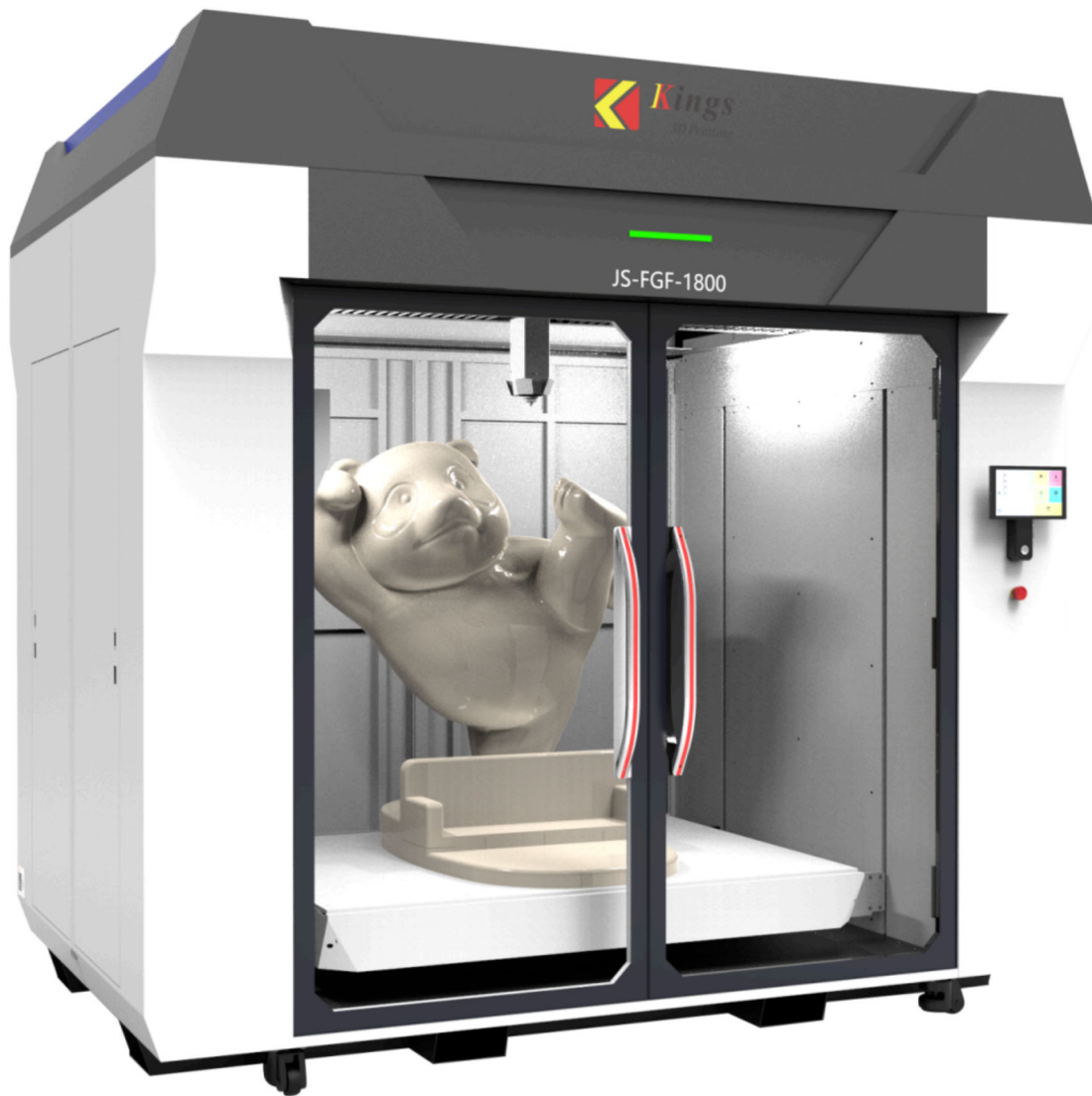
高分子颗粒打印机FGF-1800
